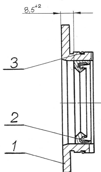
Муфта уплотнительных колец с кольцами
