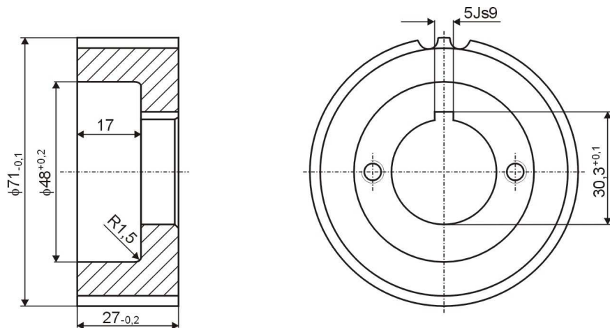
Зубчатое колесо коленчатого вала
