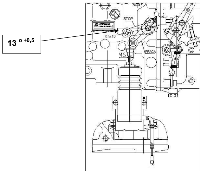
Рисунок сервомотора STOP на инжекционном насосе Motorpal
