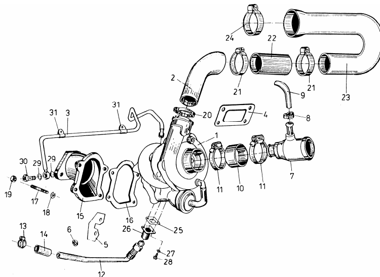
Турбокомпрессор
