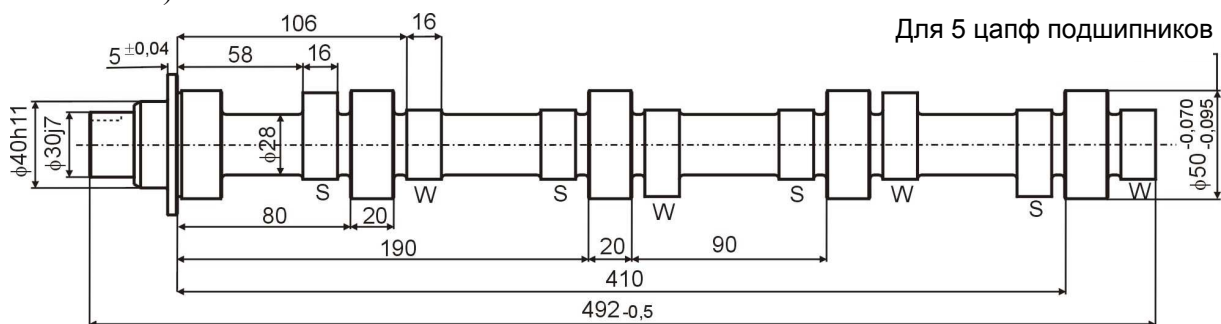
Рисунок распределительного вала
