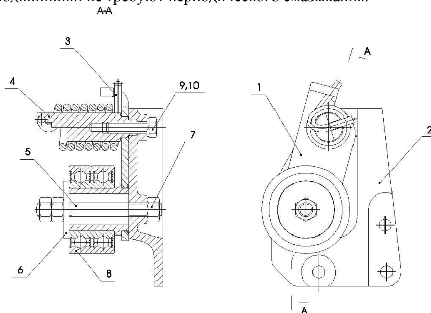
Натяжное устройство зубчатого ремня
