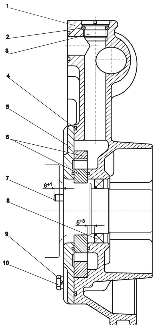
Рисунок масляного насоса
