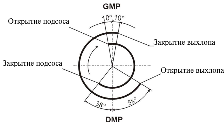
Рисунок распределительного вала
