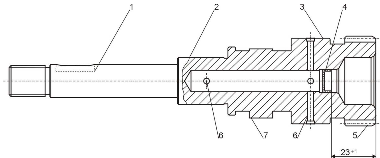
Валик привода инжекционного насоса
