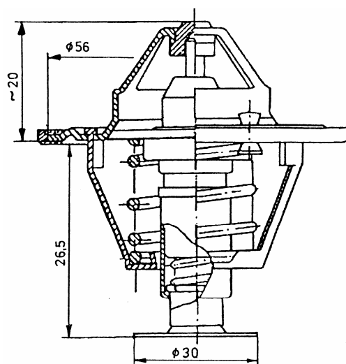
Рисунок термостата
