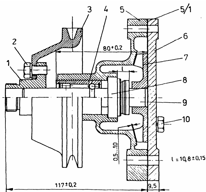
Рисунок насоса охлаждающей жидкости с ременным колесом
